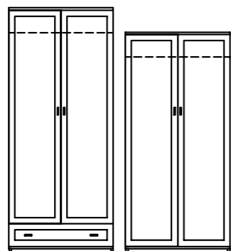
szafa Borneo BO005/BO006 wys.: 200cm, szer.: 90cm, gł.: 55cm wys.: 180cm, szer.: 90cm, gł.: 55cm
