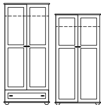
szafa Exclusive EX003/EX004 wys.: 200cm, szer.: 94cm, gł.: 55cm wys.: 180cm, szer.: 94cm, gł.: 55cm
