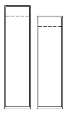
szafa Loft LO006/LO009 wys.: 200cm, szer.: 45cm, gł.: 55cm wys.: 180cm, szer.: 45cm, gł.: 55cm
