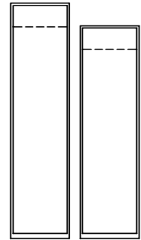
szafa Thaiti High TI002/TI003 wys.: 200cm, szer.: 45cm, gł.: 55cm wys.: 180cm, szer.: 45cm, gł.: 55cm
