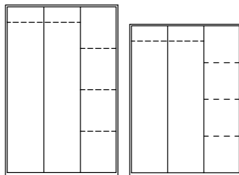
szafa Thaiti TI006/TI007 wys.: 200cm, szer.: 135cm, gł.: 55cm wys.: 180cm, szer.: 135cm, gł.: 55cm
