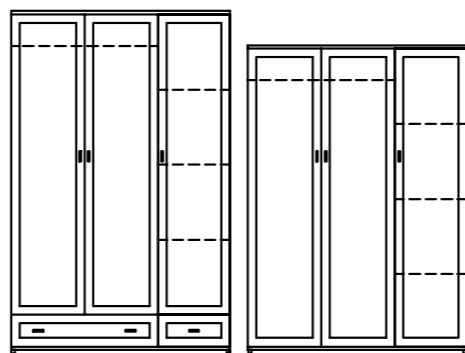
szafa Borneo BO007/BO008 wys.: 200cm, szer.: 135cm, gł.: 55cm wys.: 180cm, szer.: 135cm, gł.: 55cm
