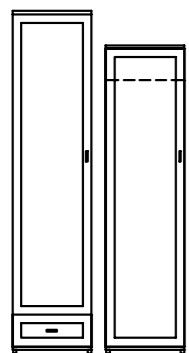
szafa Borneo BO003/BO004 wys.: 200cm, szer.: 45cm, gł.: 55cm wys.: 180cm, szer.: 45cm, gł.: 55cm
